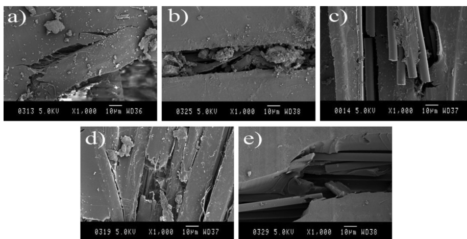
Fig. 4. SEM micrographs of (a) FlaxCP (b) FlaxCP–Carbon (c) Carbon (d) FlaxUD (e) FlaxUD–Carbon.
